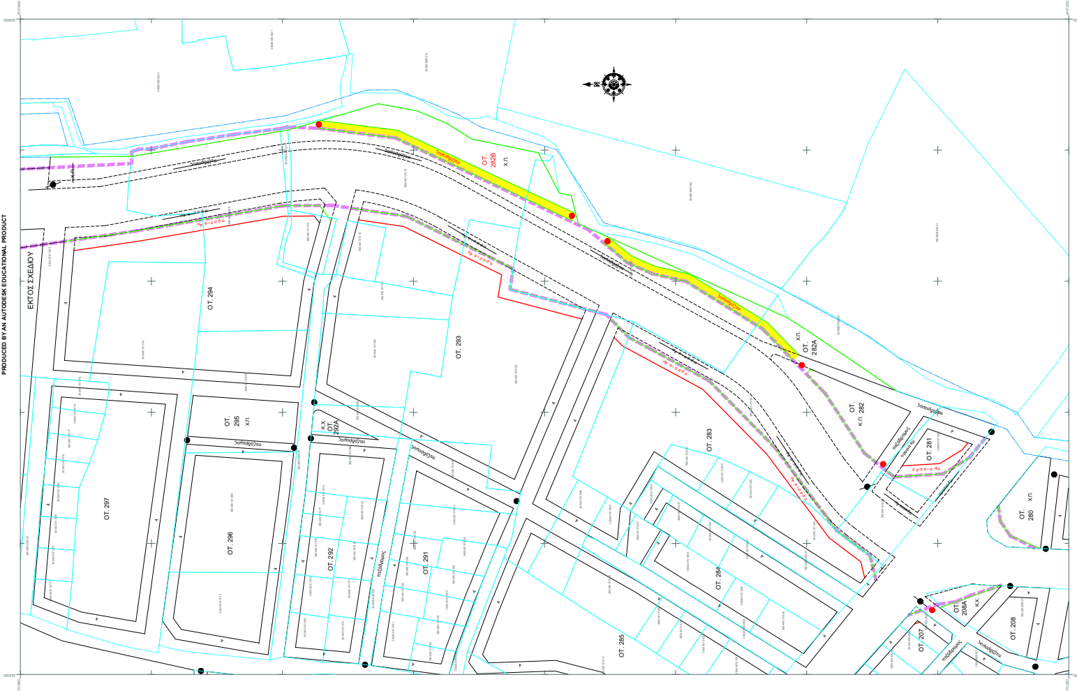
ΑΠΟΤΥΠΩΣΗ ΕΓΚΕΙΜΕΝΟΥ Π.Σ. ΑΣΤΡΟΧΩΜΑΤΟΣ ΔΗΜΟΥ ΚΑΛΑΜΑΤΑΣ ΚΑΜΑΚΑ: 1: 1000
